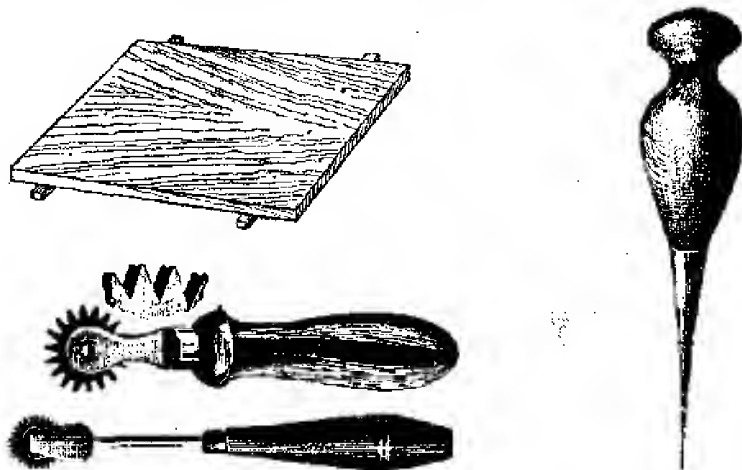
Прибор за утапање жице у саће: даска-подметач, амерички жврк за хладно утапање жице у саће, доле немачки жврк и десно шило за бушење рупа
